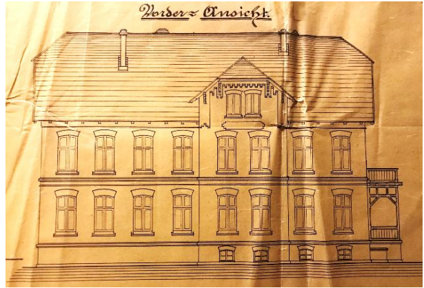
Teil der Bauzeichnung
